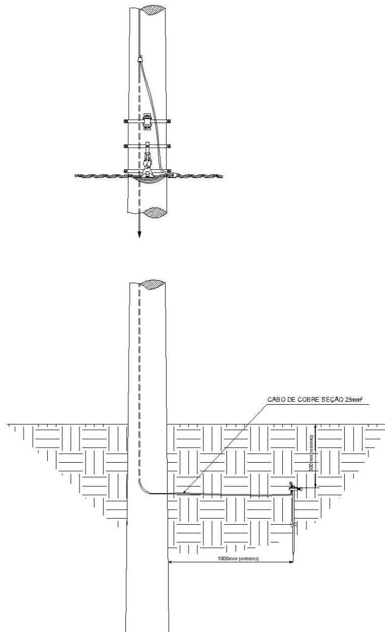
Figura 21 - Aterramento - Neutro
