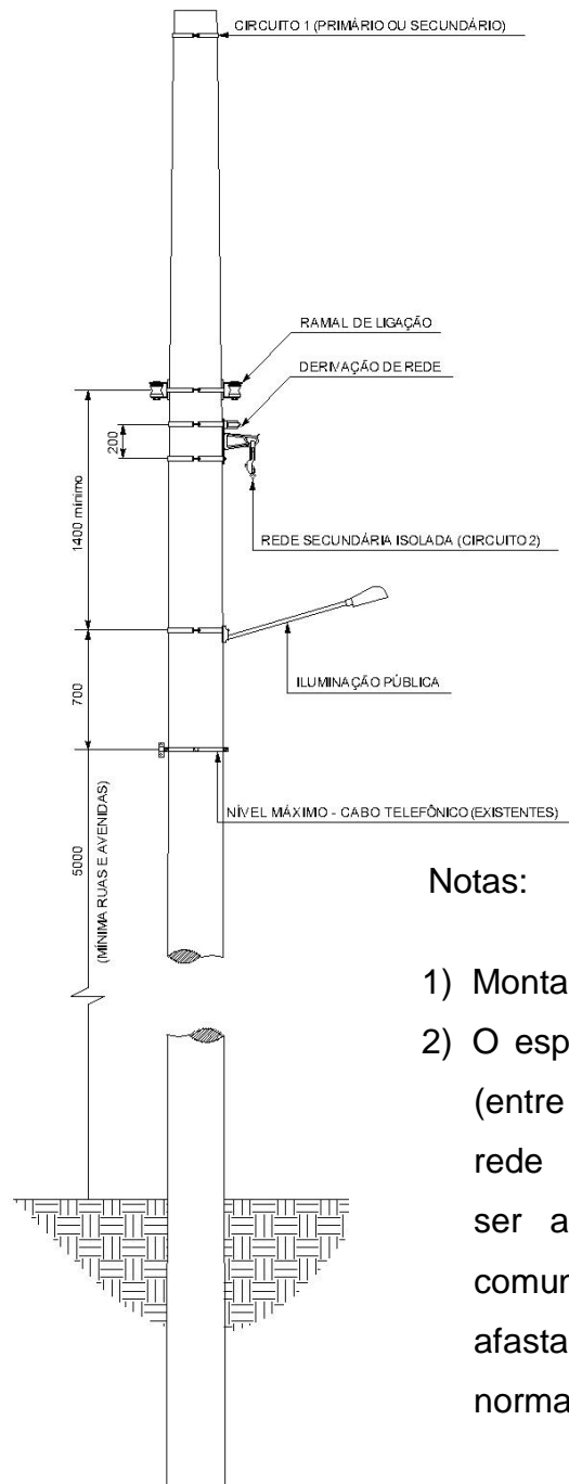
Figura 1 – Instalação básica
